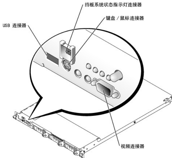
图 B-1. 前面板 I/O 端口和连接器
