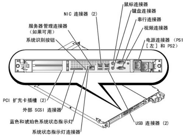
图 1-4. 背面板部件和指示灯
