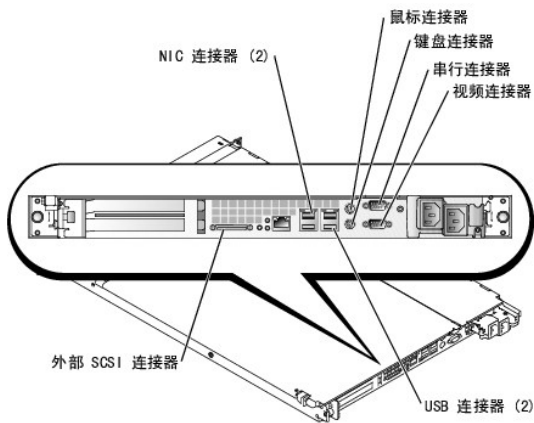
图 B-2. 后面板 I/O 端口和连接器
