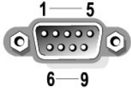
图 B-3. 串行端口连接器的插针编号
